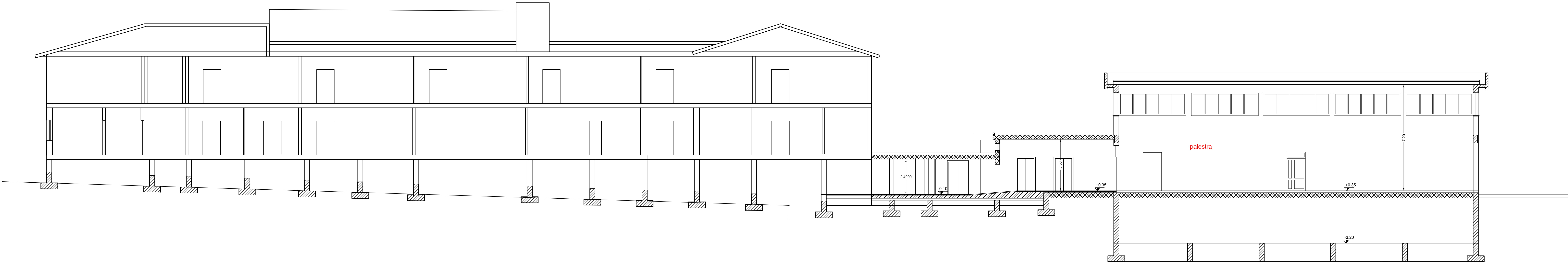
SEZIONE B-B
