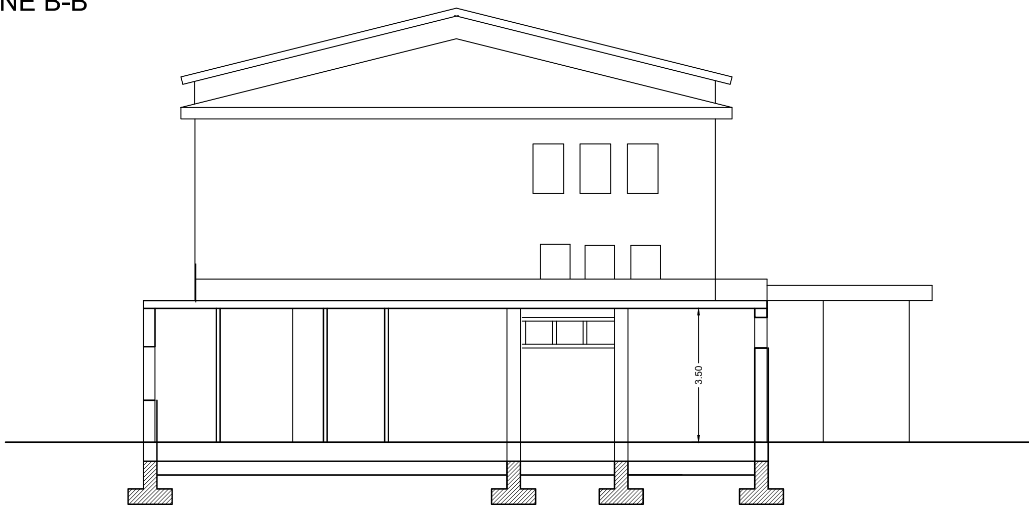
SEZIONE B-B
