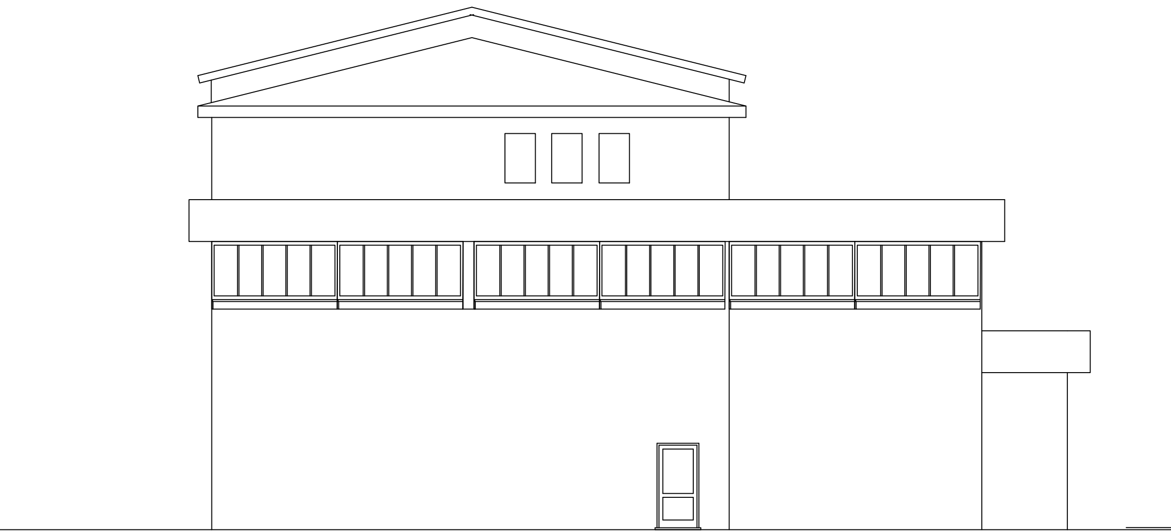
PROSPETTO NORD
